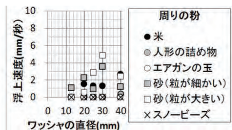
図12 模擬ナッツ(座金)の浮上速度
