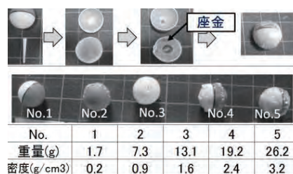
図6 重さの異なる模擬ナッツ(浮き)
