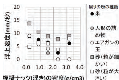
図7 模擬ナッツ(浮き)の密度と浮上速度の関係
